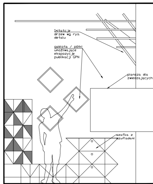
PRZEKRÓJ DD 1/50
